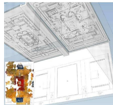
Assonometria ricostruttiva dell'ambiente dipinto. Uno dei soffitti
